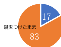
バイク (%)
