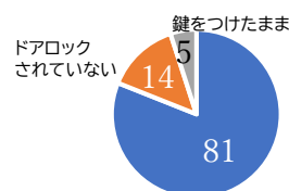
バイク (%)
