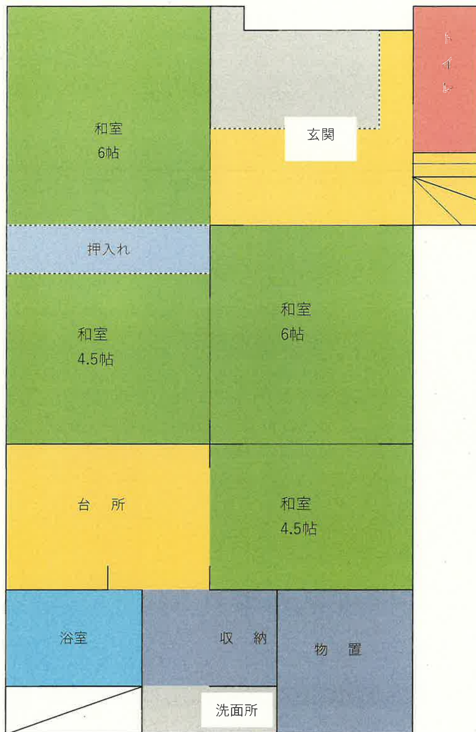
1 階平面図
